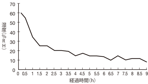
庫内湿度の測定例
